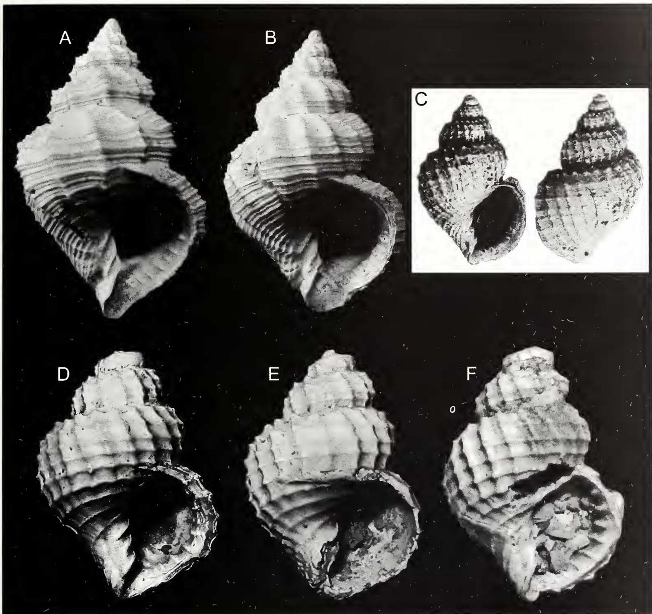
Fig. 6. A, B. Bonellitia striatissima n. sp. A Cava Campore (Parma), Piacenziano, H = 18,5 mm (coll. Della Bella). B Cava Campore (Parma), Piacenziano, H = 18,4 mm (coll. Della Bella). C. Bonellitia chainei (Peyrot, 1928), da Peyrot (1928, modificata), H = 11,5 mm. D-F. Bonellitia sp. D Rio Merli (Ravenna), Piacenziano, H = 6,5 mm (coll. Brunetti). E. Cava Campore (Parma), Piacenziano, H = 7 mm (coll. Brunetti). F. Cava Campore (Parma), Piacenziano, H = 7,8 mm (coll. Brunetti).
